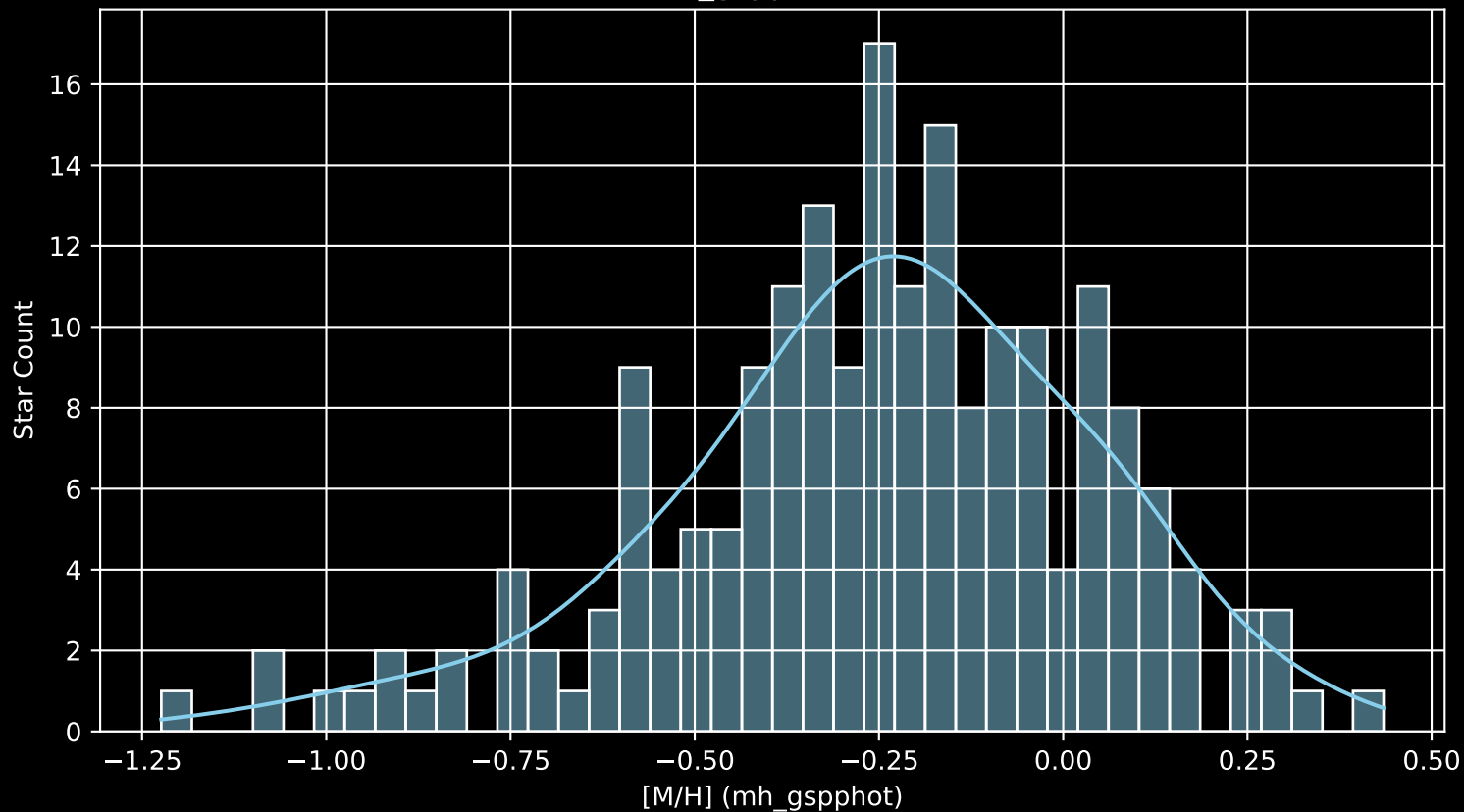
GALAH DR4 Field: [7187] [M/H] (mh_gspphot) (n= 197)
