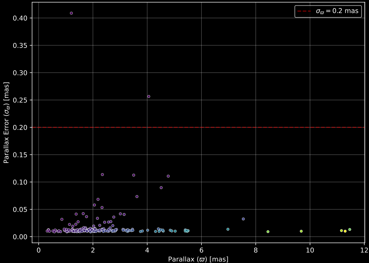
GALAH DR4 Field: [7187] Parallax Quality (n= 198)
