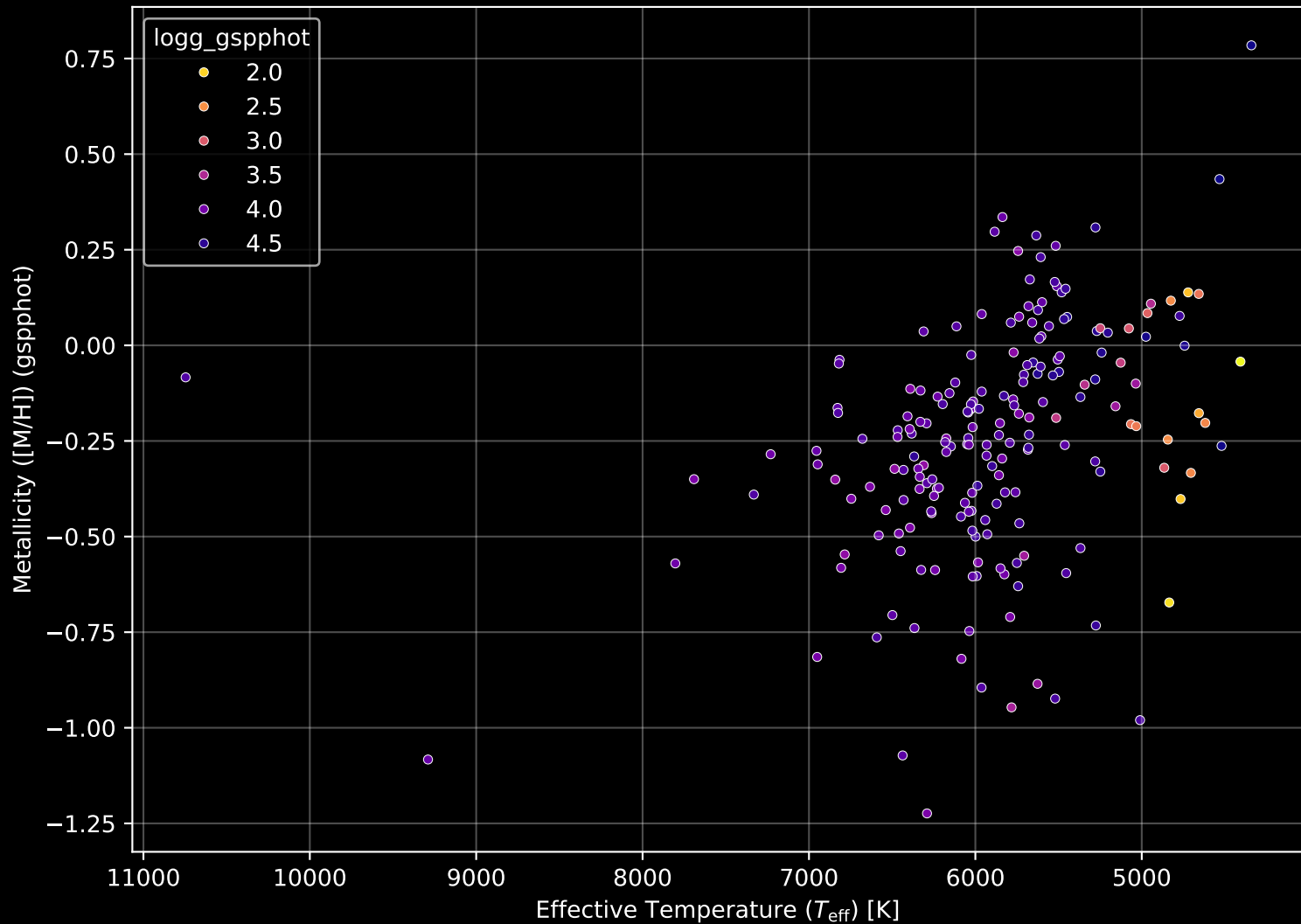
GALAH DR4 Field: [7187] Stellar Population Parameters (n= 198)
